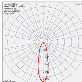
36° FWHM TIR
